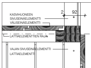
Detaili: väliseinän aseointi 1:5
