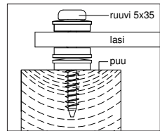
Detalji: lasin kiinnitys
