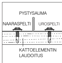
Detailji 1:2
