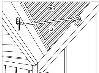
Detaljritning för fastsättning av trådhasan
