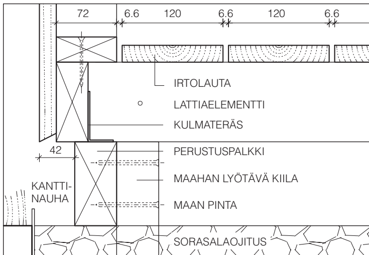
Detalji 1: perustusten asemointi 1:5
