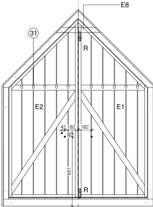
Projektiokuva takaa päätelementistä
