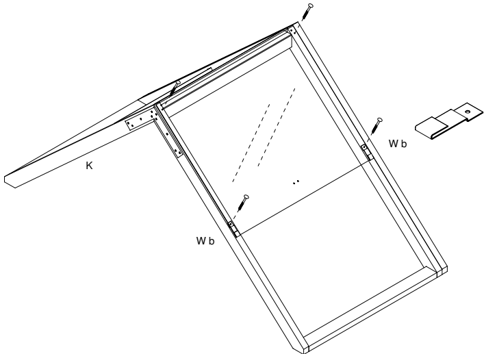
Detailji: lasin kiinnitys
