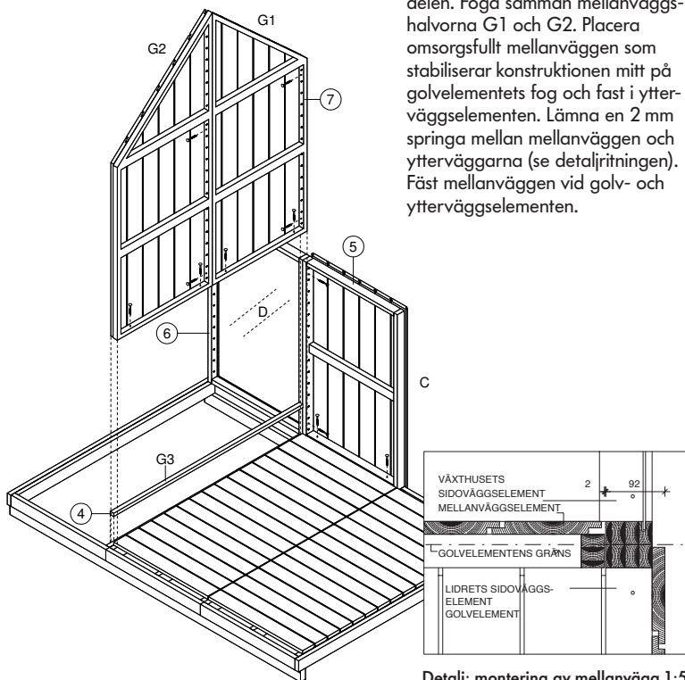
Detalj: montering av mellanvägg 1:5
