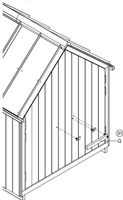
Detaljritning för fastsättning av trådaken.
