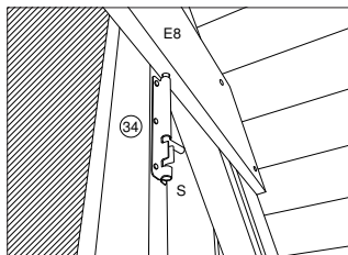
Detalji työntösälvan kiinnityksestä
