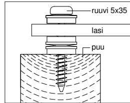
Detailji: lasin kiinnitys
