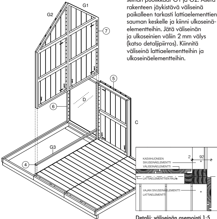
Detalji: väliseinän aseointi 1:5
