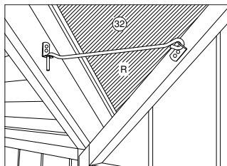
Detaljritning för fastsättning av trådaken.
