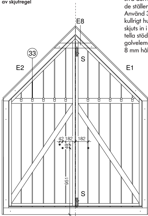
Projektionsbild av gavelementen bakifrån
