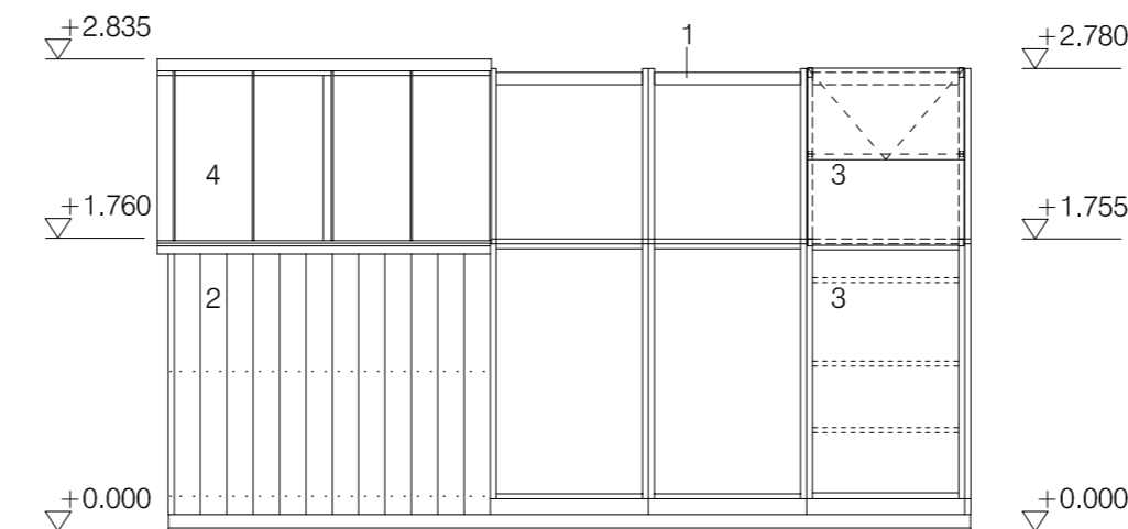
SIVUJULKISIVU
