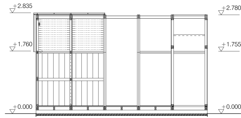
PITUUSLEIKKAUS C-C
