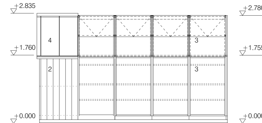
SIVUJULKISIVU
