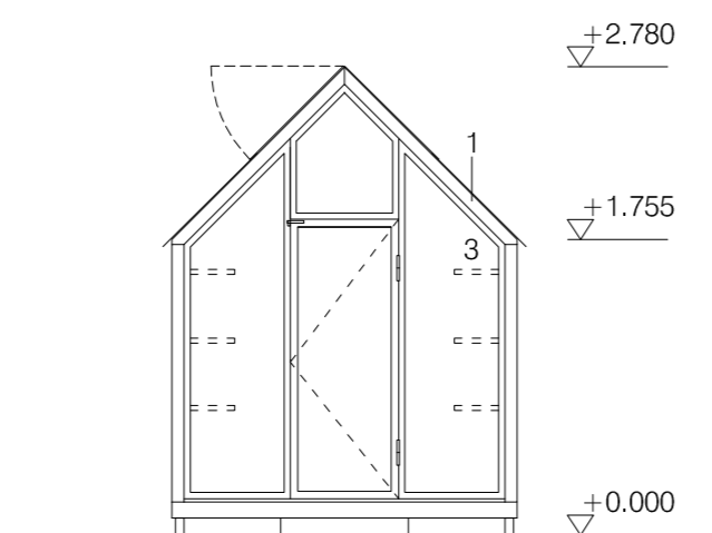
KASVIHUONEEN PÄÄTYJULKISIVU
