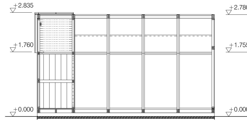
PITUUSLEIKKAUS C-C
