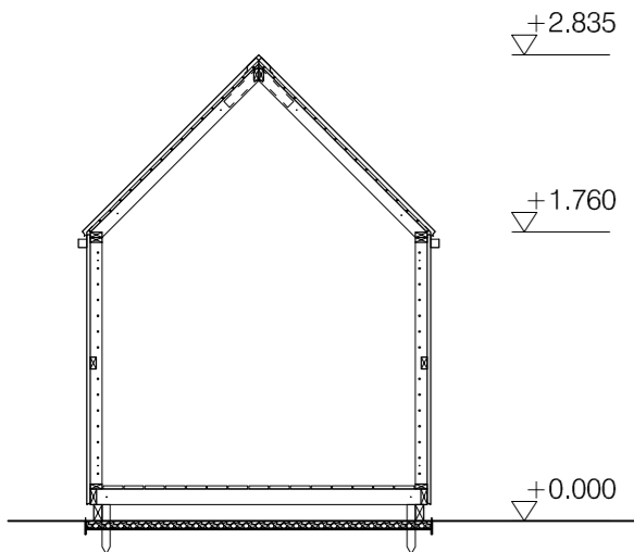
LEIKKAUS A-A VAJAN KOHDALTA
