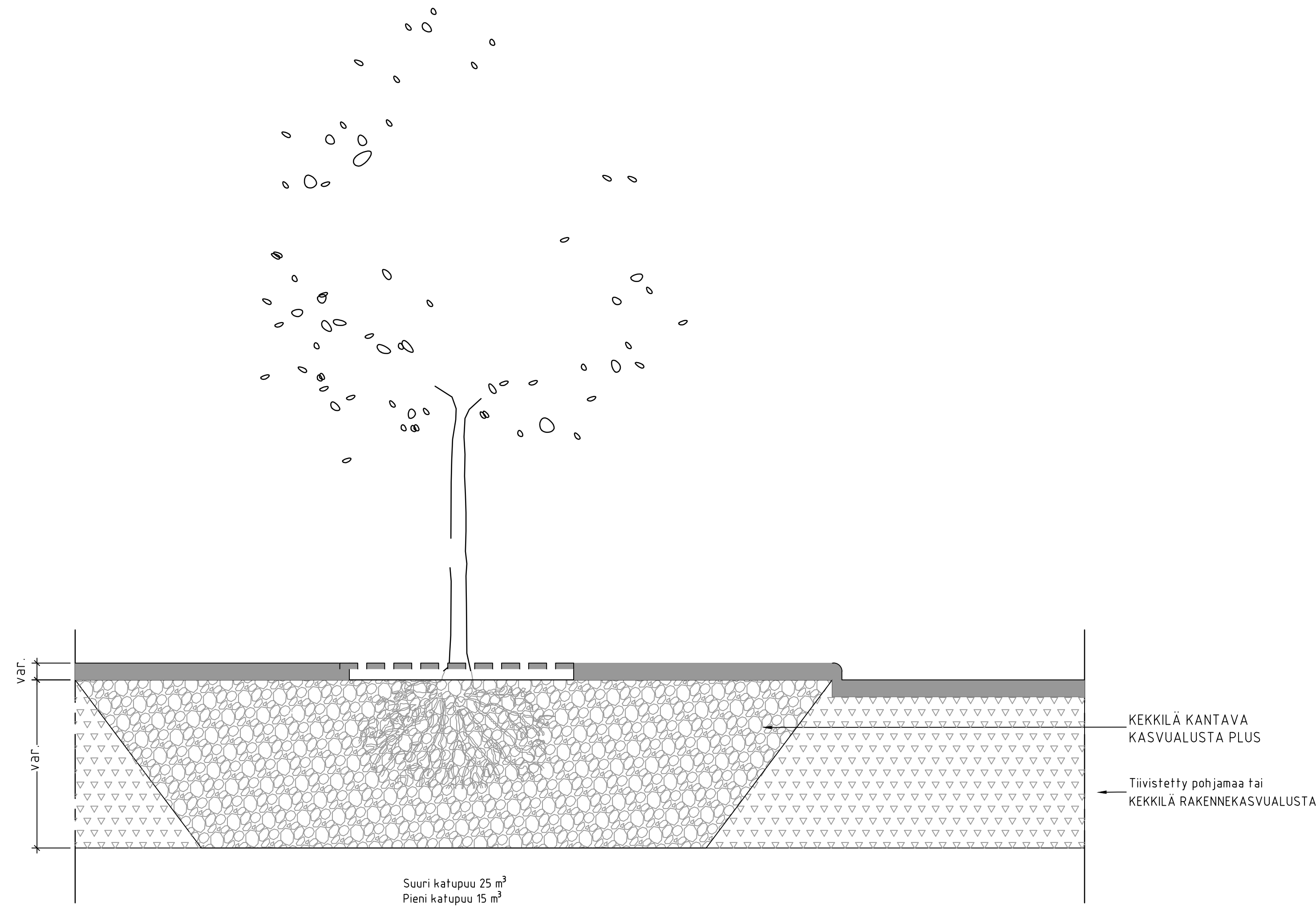
KATUPUUT LIIKENNEALUEILLA KEKKILÄ KANTAVA KASVUALUSTA PLUS RAKENNELEIKKAUS, MITTAKAAVA 1:20/A1. Kaikki mitat millimetriä (mm)
